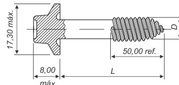
Rosca modelo B
