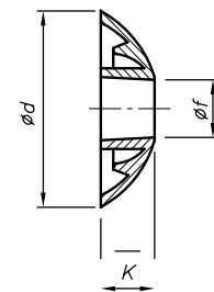
Arruela de Vedação
